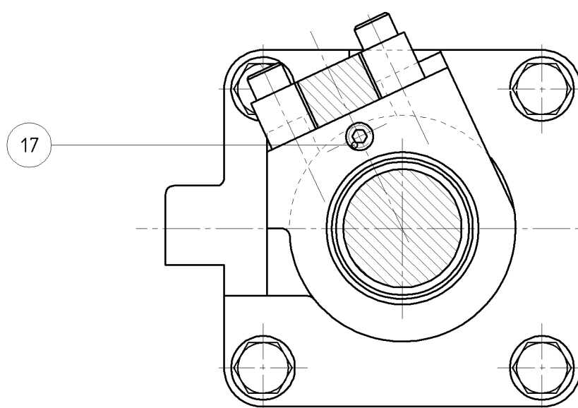
Sezione parziale "B-B"
