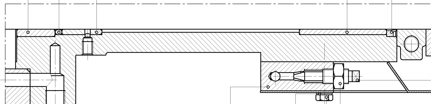
Sezione parziale "A-A"
