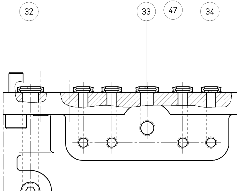
Vista parziale "Z"
