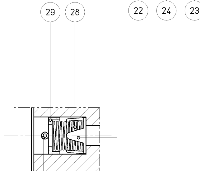
Sezione parziale "A-A"
