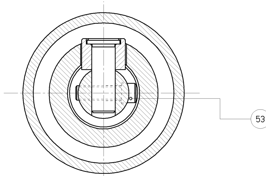
Sezione "C-C"
